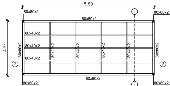
Estructura Piso
