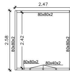
Corte 1-1
