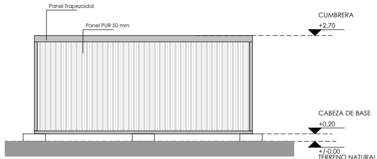
Vista Posterior
